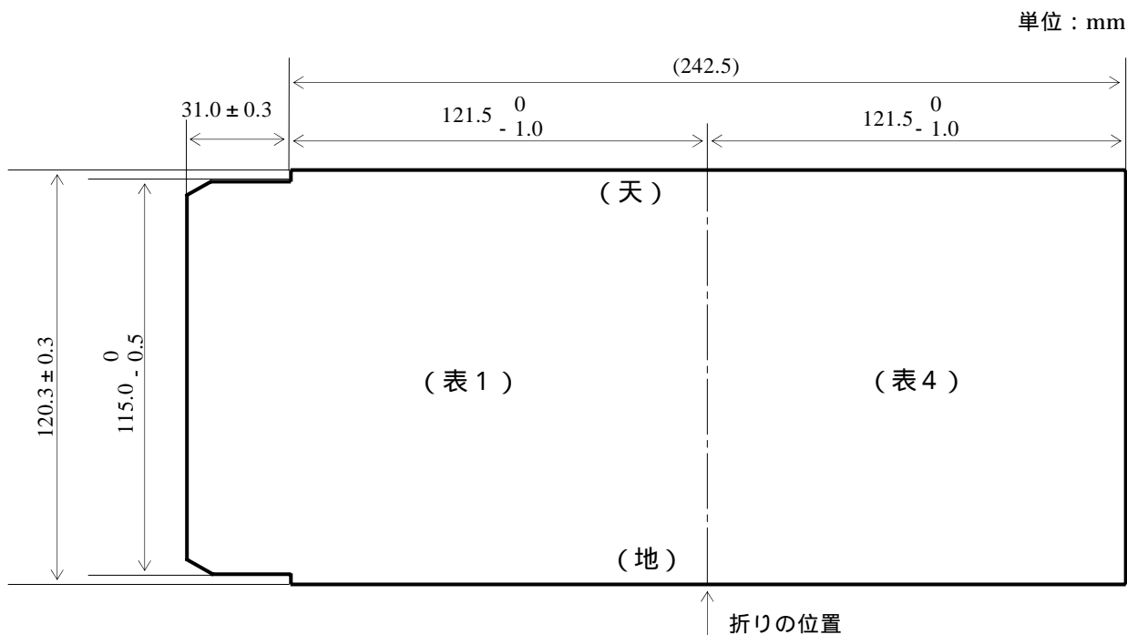
図7 型の展開図
