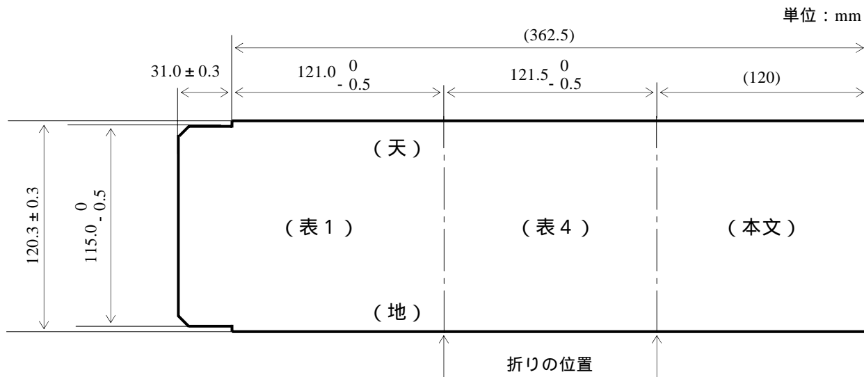
図 8 型の展開図
