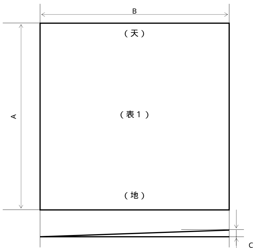
図1 ジュエルケース用表カードの形状(型、型、型共通)
