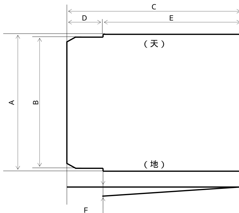
図5 マキシケース用表カードの形状（型、型、型共通）
