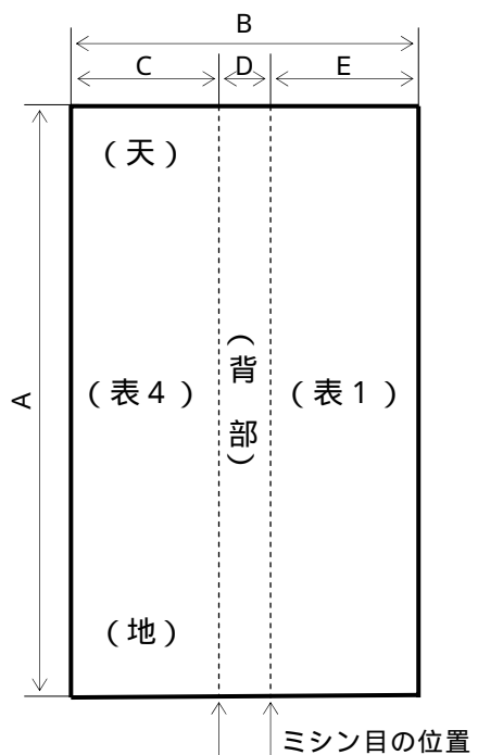
図 13 キャップの形状
